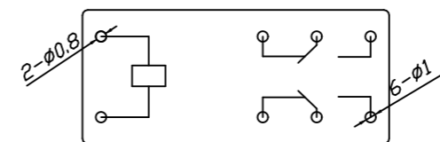
电气原理图
