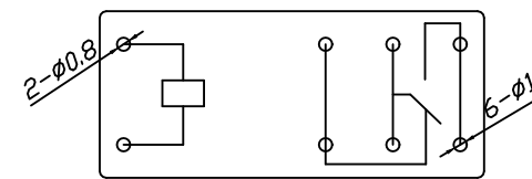
电气原理图
