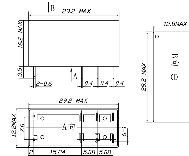
外形安装尺寸图
